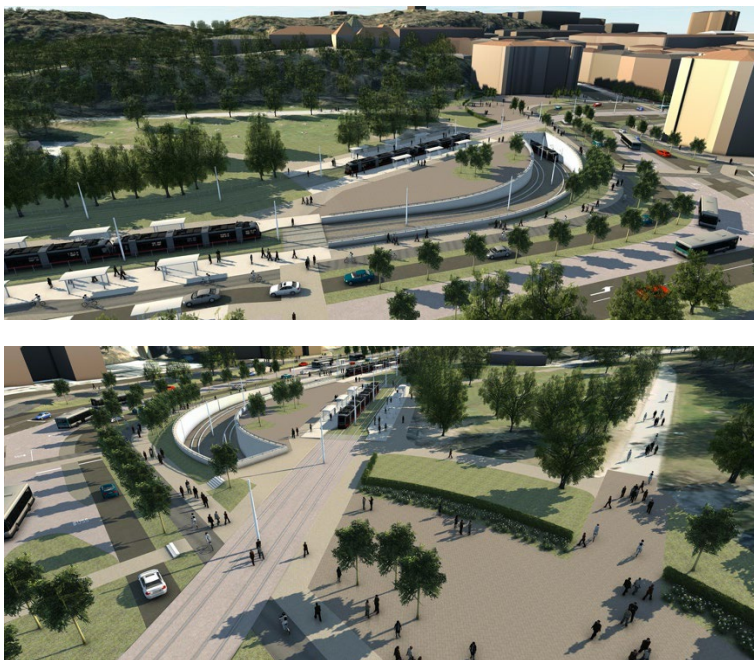
Visionsbilder Hållplats Linnéplatsen. Trågets fria utrymme utgörs av en bottenplatta och två väggar. Längden på den södra trågväggen vid Linnéplatsen är ca 89 meter och höjden varierar från 0,6 till 5,1 meter. Arealen är totalt ca 240 m 2 . Den norra trågväggen är ca 113 meter och höjden varierar mellan 0,6 och 5,1 meter. Arealen är totalt ca 248 m 2 .
